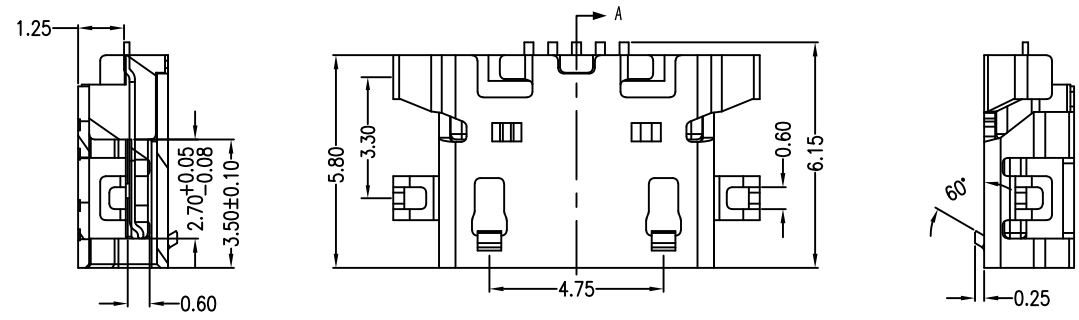
SEC A-A
